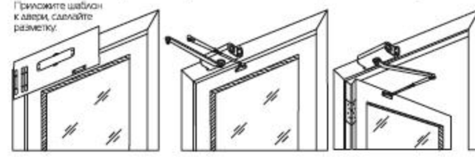
Вар.2 Верхняя установка для правой двери
