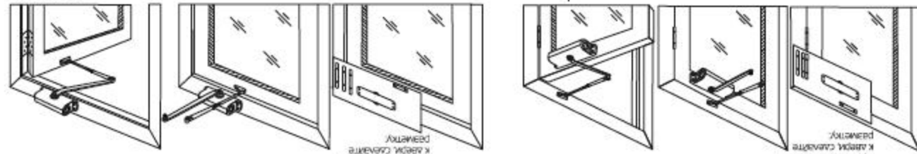
Вар.3 Стандартная установка для правой двери
