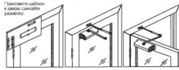
Вар.1 Стандартная установка для левой двери
